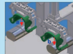
a. 熱壓狀態 Hot creasing b. 冷壓狀態 Cold creasing
